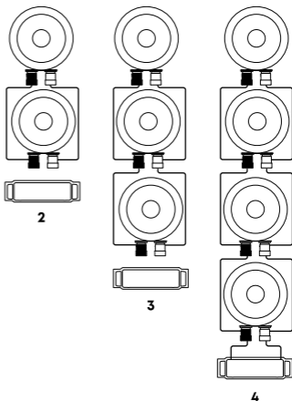
Последовательное подсоединение
