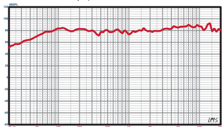
График АЧХ TENOR T 52
