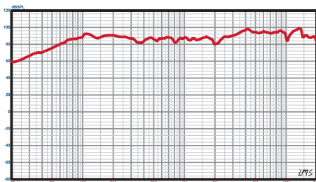
График АЧХ TENOR T 62
